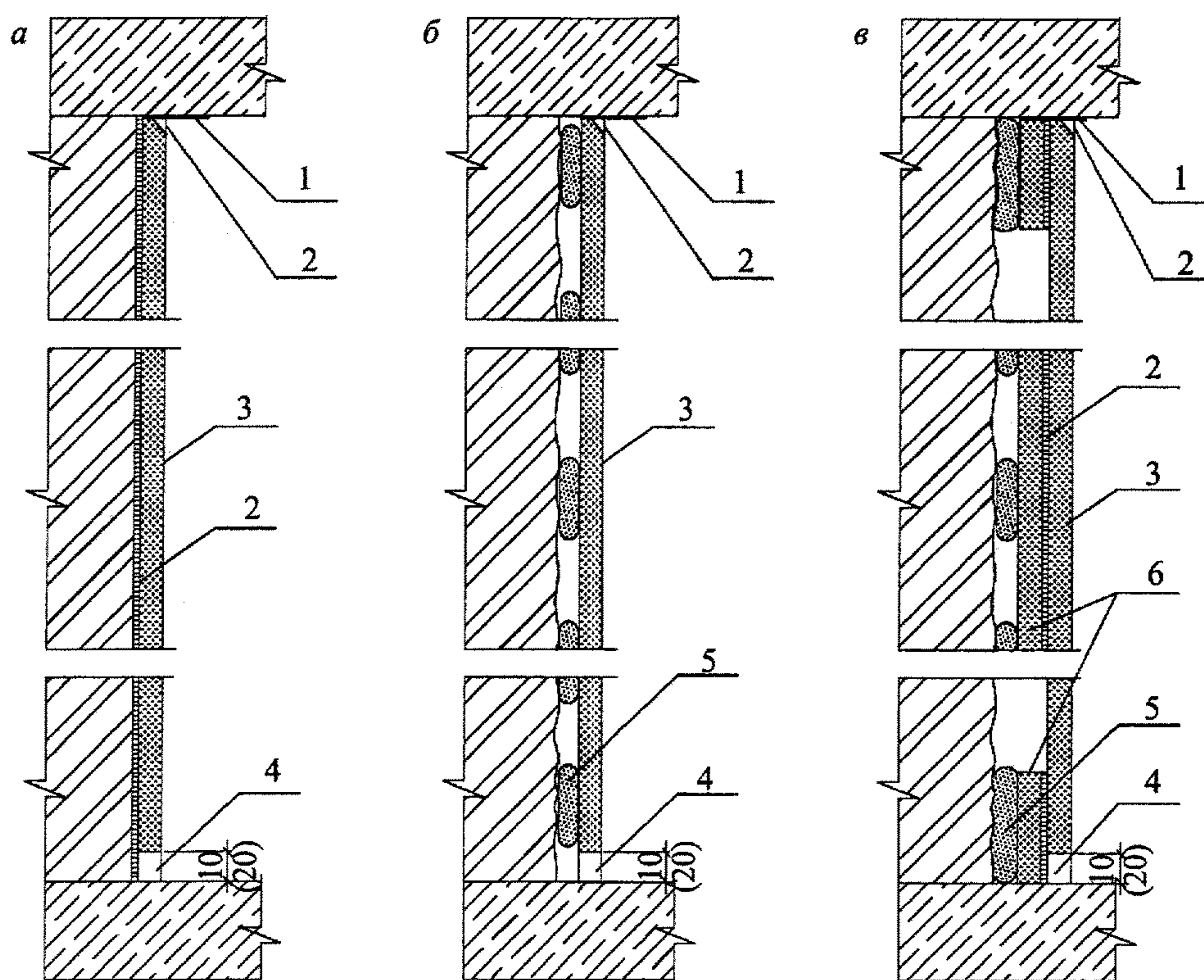
a – крепление гипсокартонных листов на ровное основание; б – крепление гипсокартонных листов на основание с неровностью до 20 мм; в – крепление гипсокартонных листов на основание с неровностью свыше 20 мм
