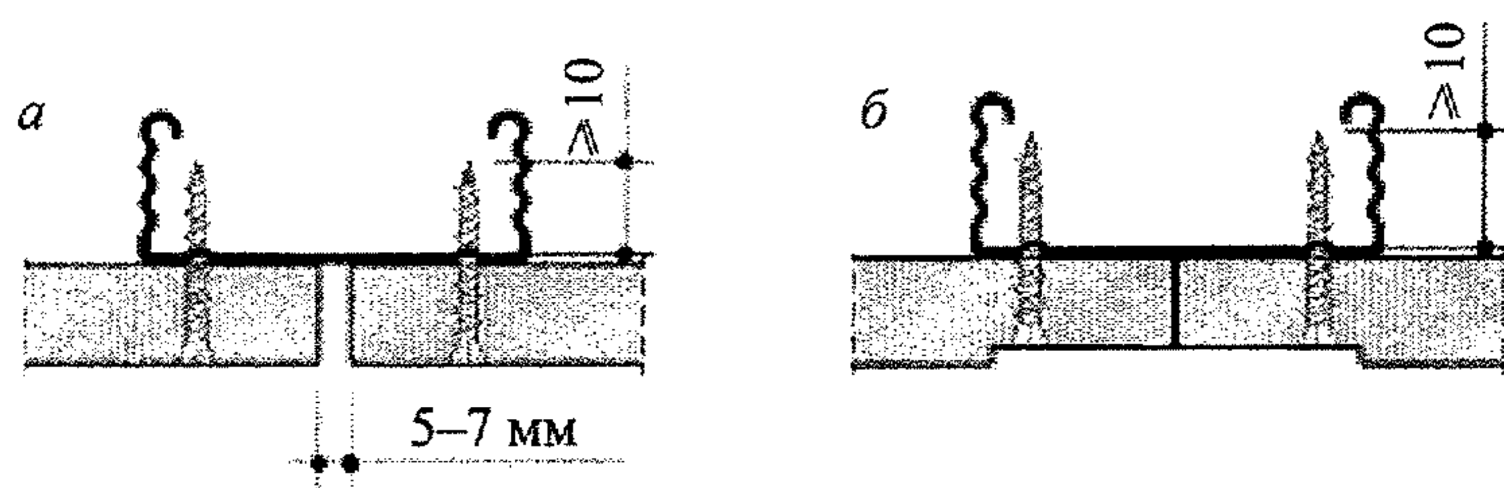
а – с прямой кромкой; б – фальцевой кромкой
