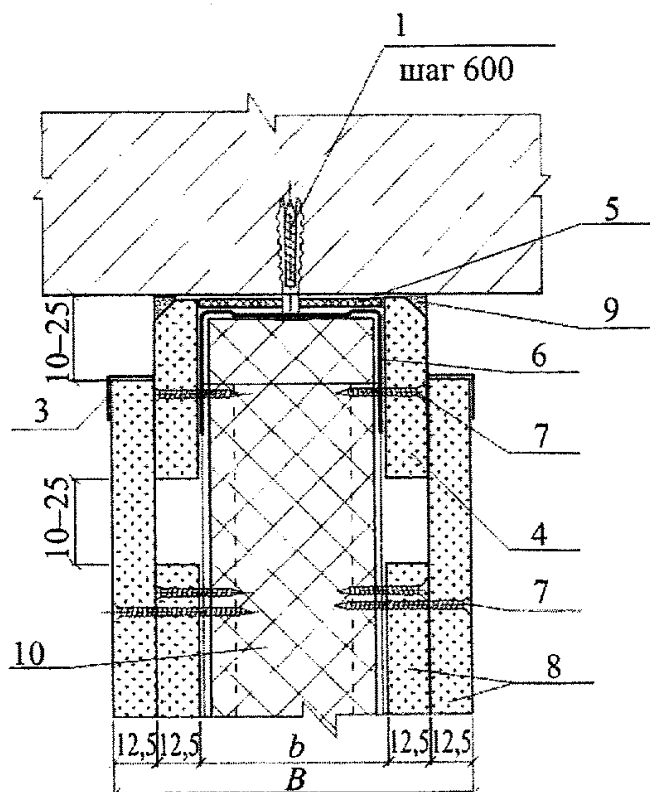
Рисунок 3 – Присоединение перегородки с обшивками из гипсокартонных или гипсоволокнистых листов к потолку
