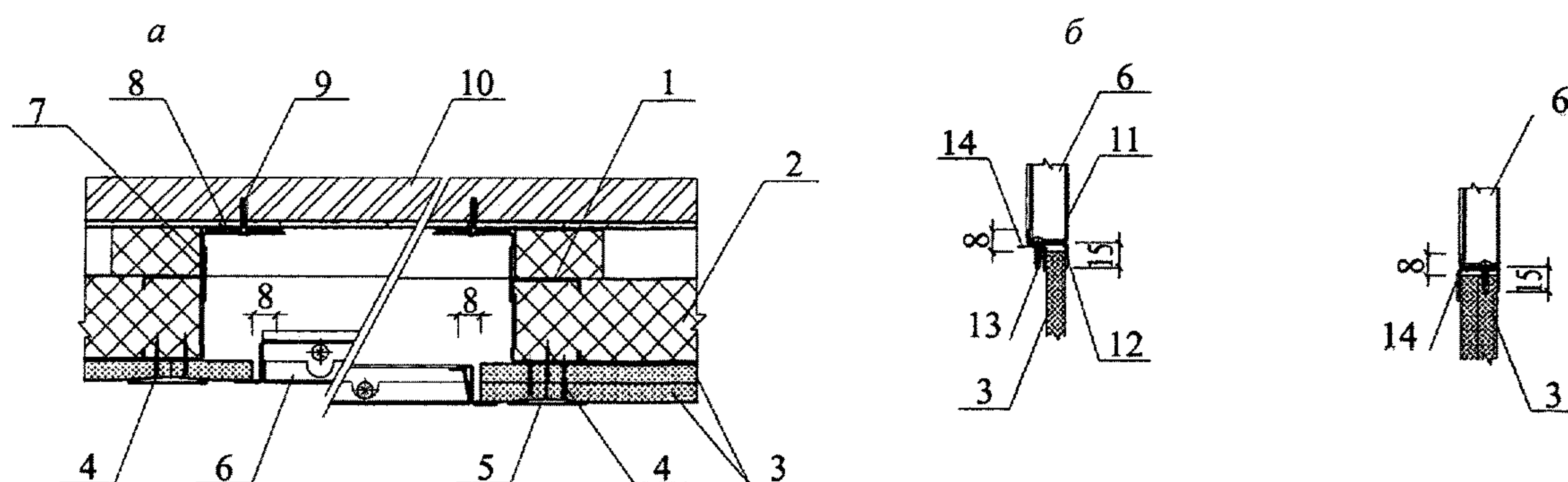
a – горизонтальный разрез; б – вертикальный разрез
