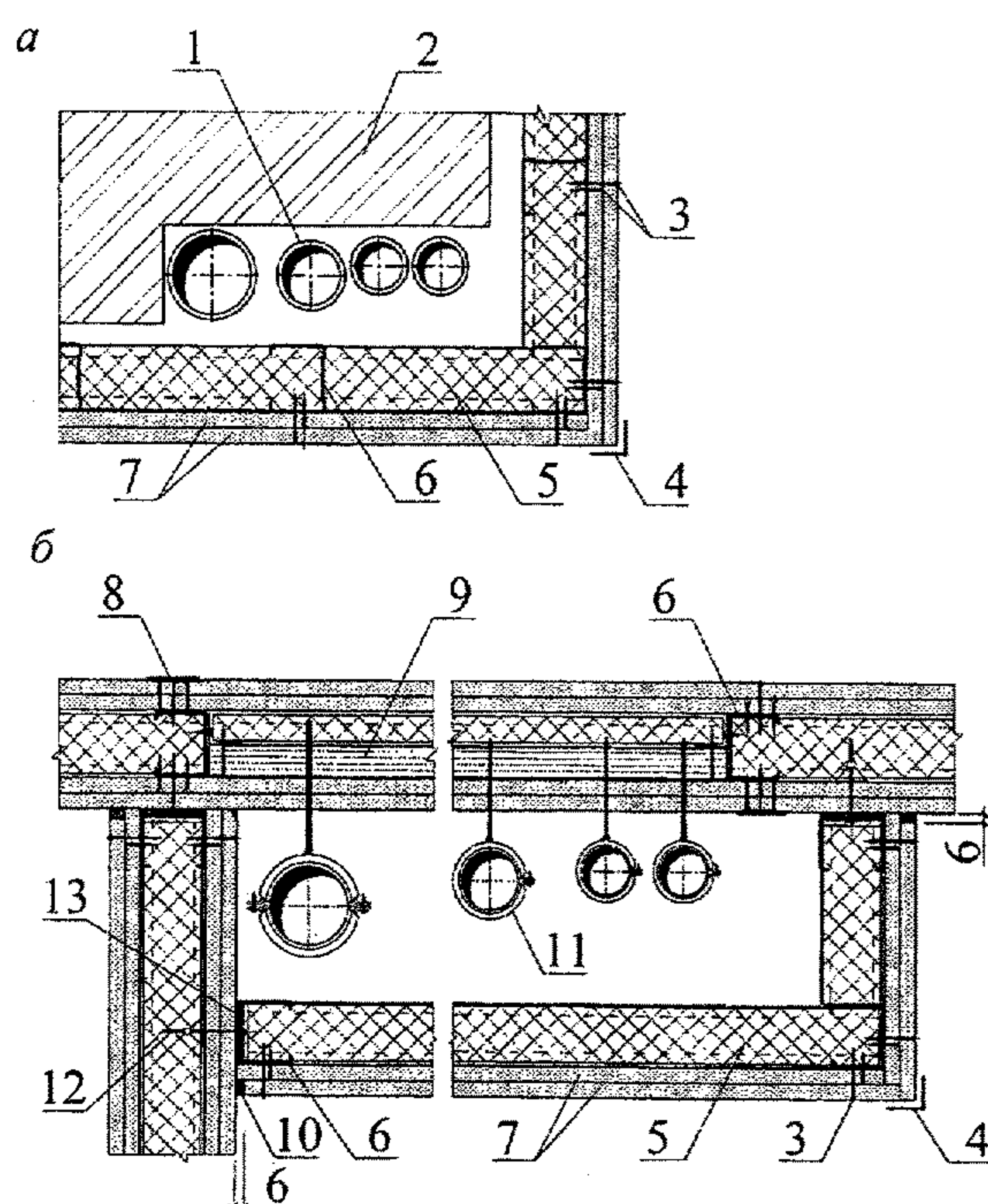
a – у несущей стены; б – у перегородки
