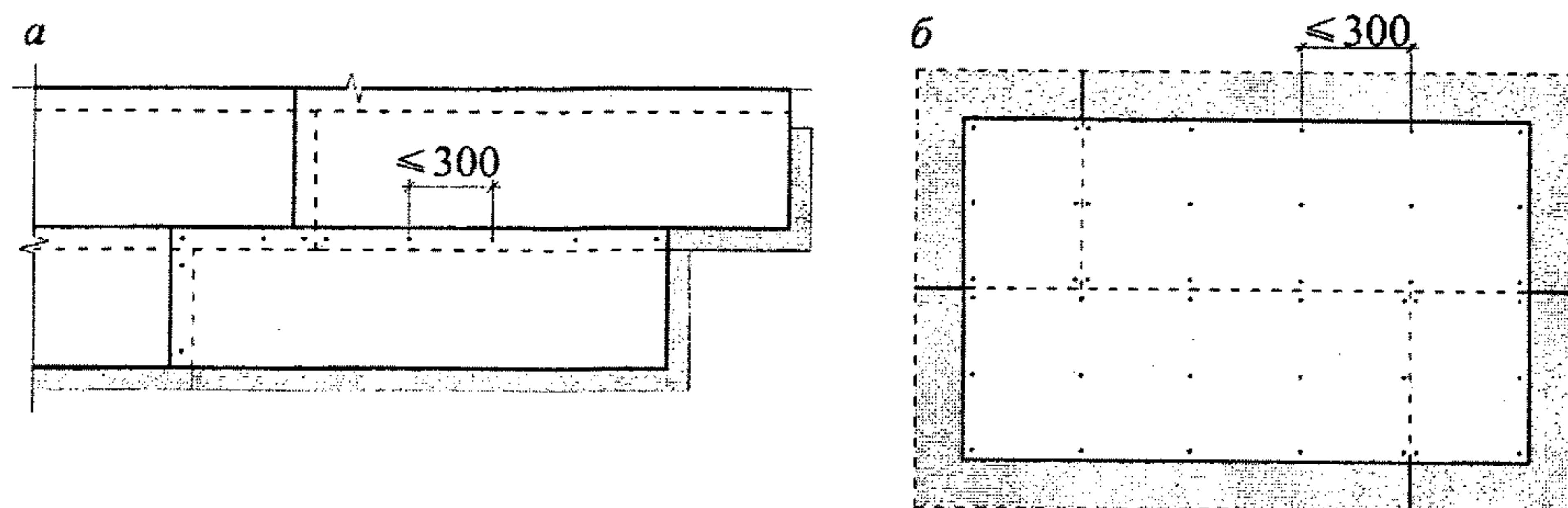
a – крепление ЭП; б – крепление малоформатных ГВЛВ
