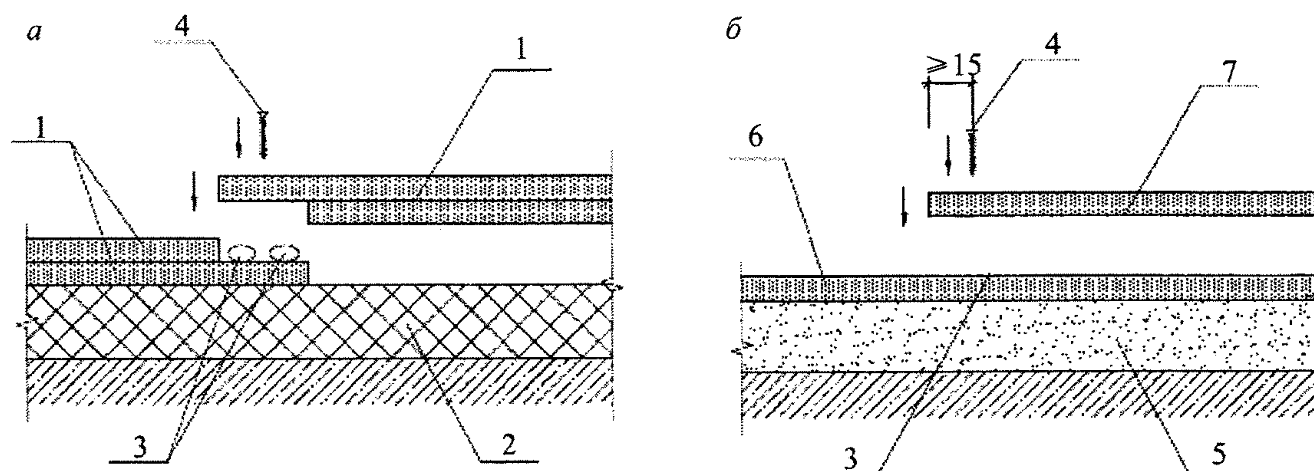
а – соединение ЭП; б – соединение малоформатных ГВЛВ
